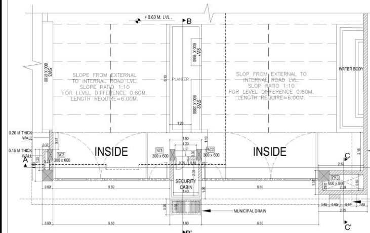
ENTRY / EXIT + 0.00 M. LVL.
